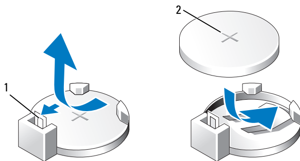
1 Leva di sblocco della pila
